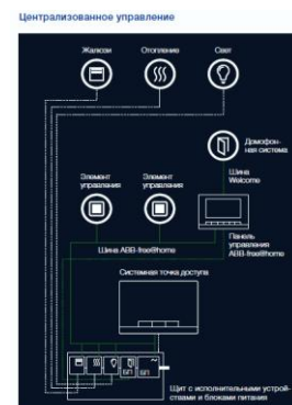
Централизованная схема подключения, с установкой исполнительных устройств на DIN-рейку
